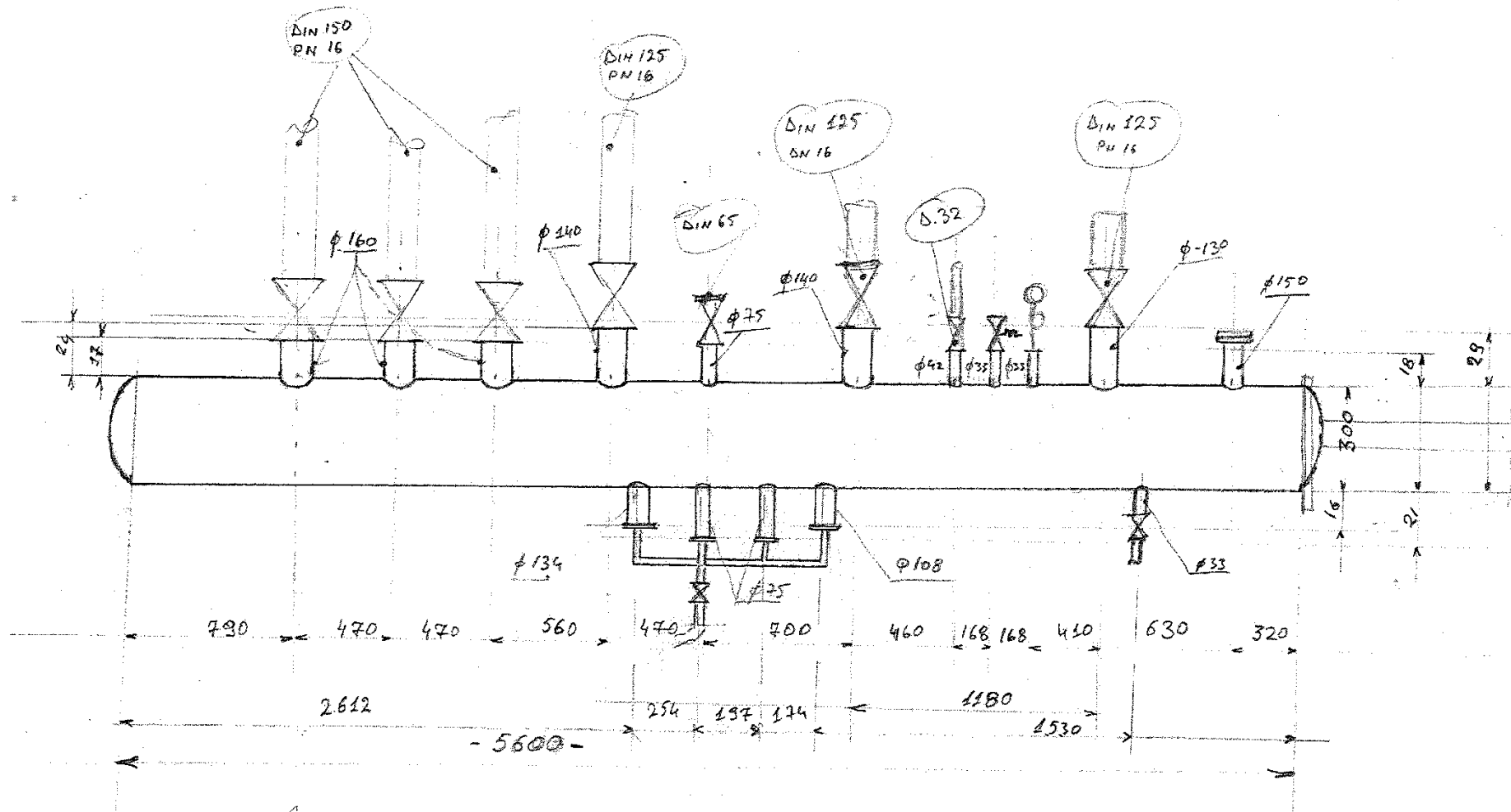
Εικόνα 1. Σκαρίφημα υφιστάμενου ατμοδιανομέα προς αντικατάσταση.
